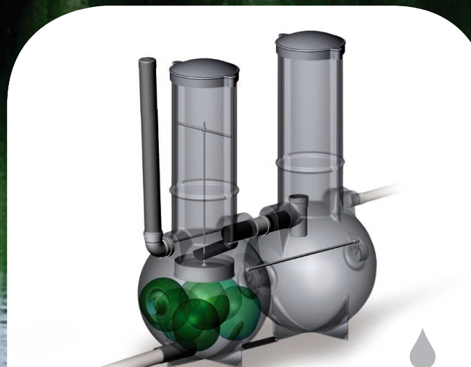
Labko® BioRami 500 0,5 m³ LVI-numero 3629 005
