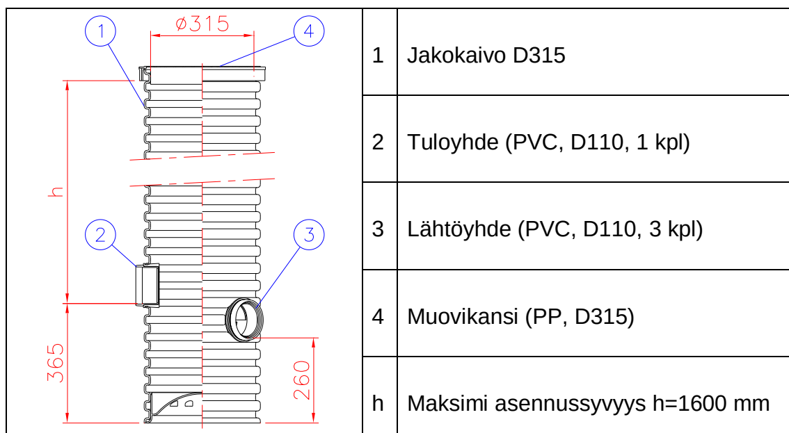
Kuva 3. Jakokaivon rakenne.
