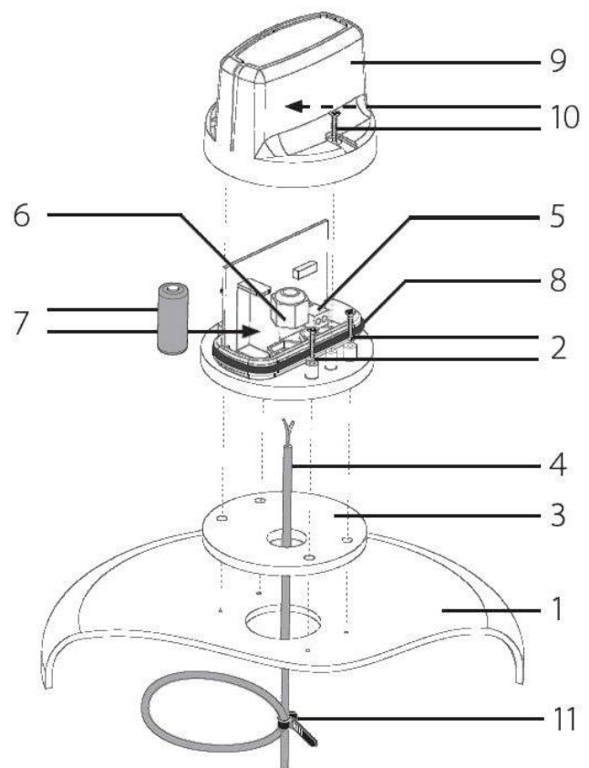
Kuva 13. Hälytinanturin asentaminen.
