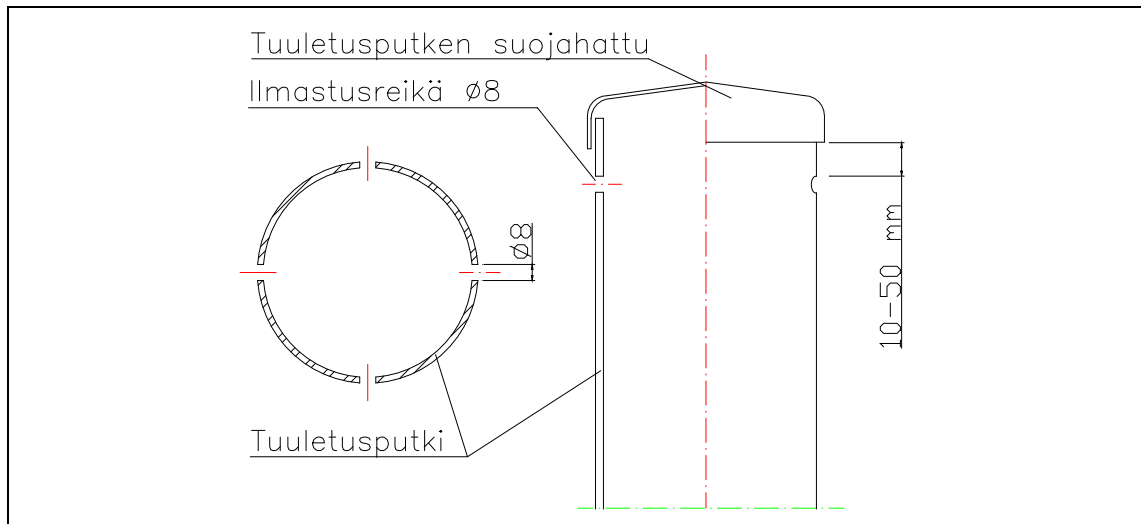
Kuva 10. Tuuletusputken ilmastusreiät.
