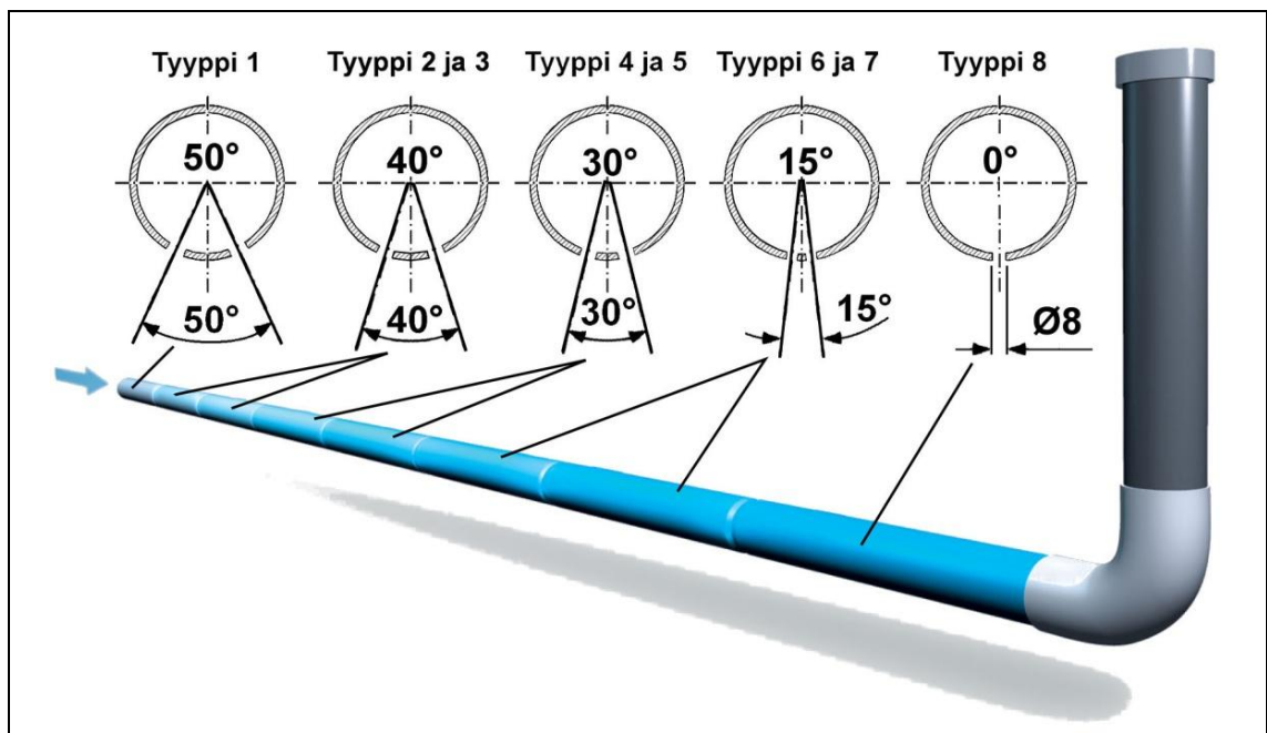
Kuva 9. Imeytysputkiston putkityypit.
